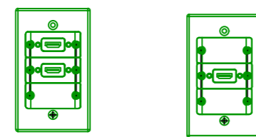
DET.1 - INTERFACES HDMI KRAMER ESC. 1:5
