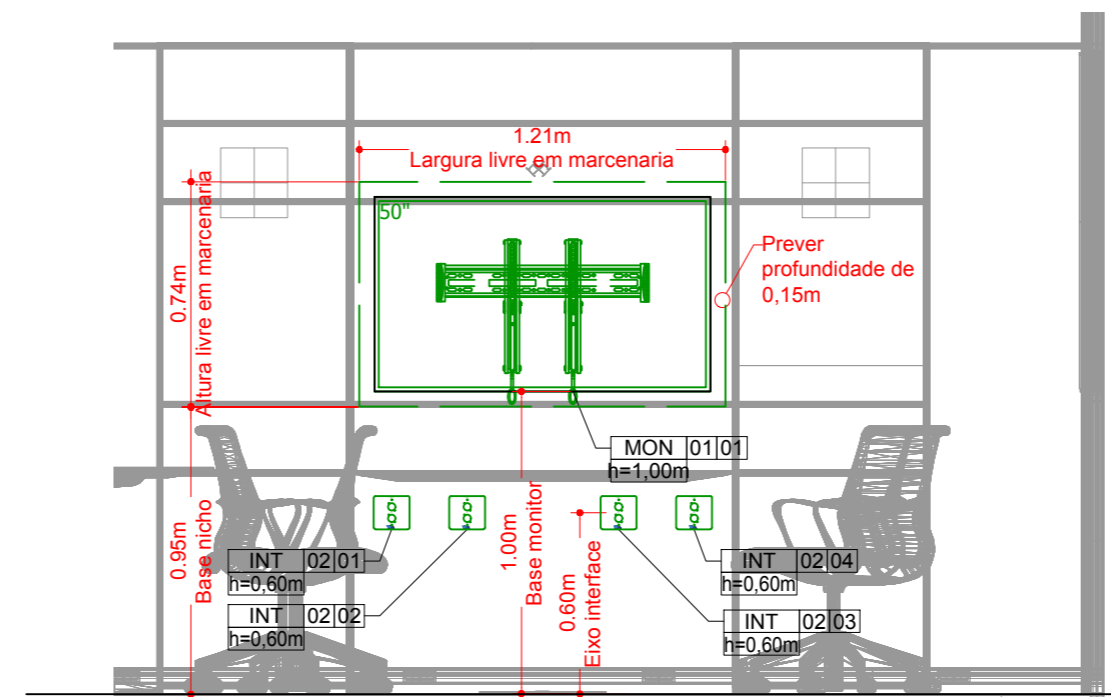
ELEVAÇÃO DE EQUIPAMENTOS 01 - ESTUDIO - 01º PAVIMENTO ESC. 1:50
