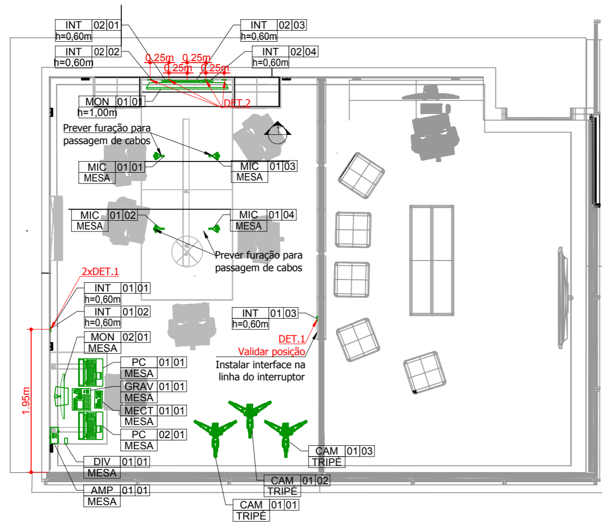
PLANTA DE LAYOUT DE PISO - ESTUDIO - 01º PAVIMENTO ESC. 1:50
